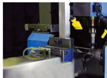
Magazine Type (輸送帶型餵料裝置)
