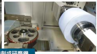
德製自動送料 - 擺線齒輪創成研磨機
