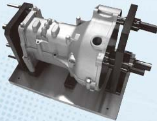
汽車變速箱孔位檢具
