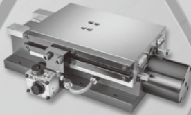
油壓滑台
