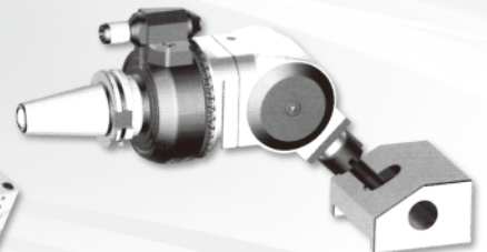
■ GERARDI 角度銼頭
