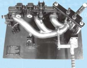
汽車排氣管綜合檢具
