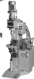
LF-168 泛用型油壓式鉚釘機 鉚合能力 Ø 3-12 mm
