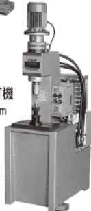
LF-188-3A 重型油壓式鉚釘機 鉚合能力 Ø 8-21 mm
